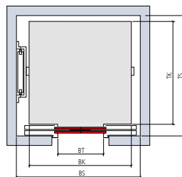
Simple accès Porte télescopique à ouverture centrale 2 vantaux
